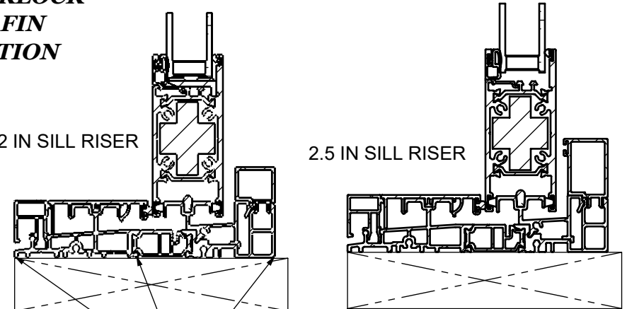
SECTION B-B SCALE 1 : 3
